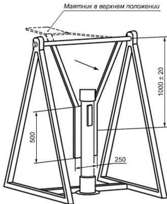
Рисунок 11 - Схема установки маятникового типа
