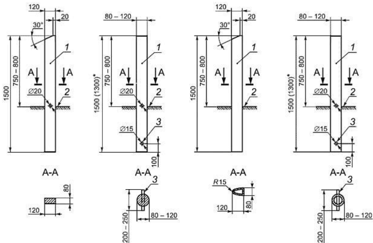
Рис.1-4. Форма и размеры сигнальных столбиков типа С1
